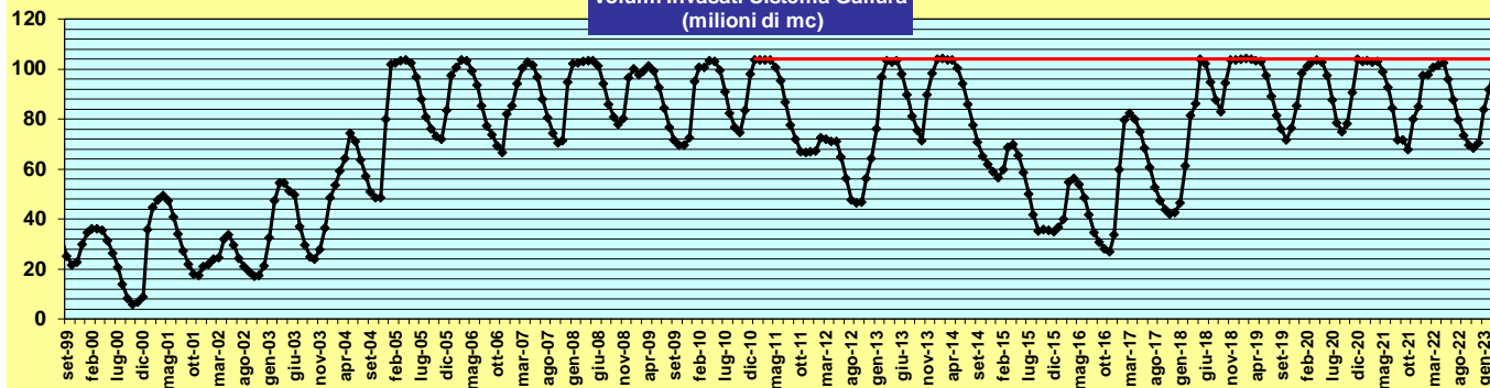
Volumi Invasati Sistema Gallura (milioni di mc)
